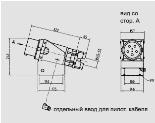
Чертеж 2 MB 197 Размеры, мм.
