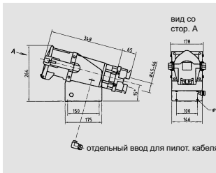
Чертеж 1 MB 385 Размеры, мм.
