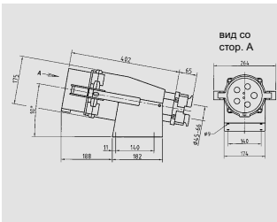
Чертеж 2 MB 200/1 Размеры, мм.
