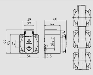
Чертеж 1 MB 27/30 Размеры, мм.
