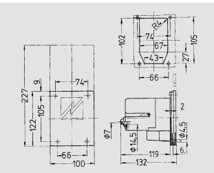
Чертеж 2 MB 70
