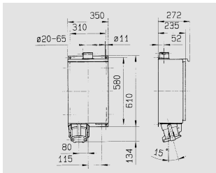
Чертеж 1 MB 387 Размеры, мм.
